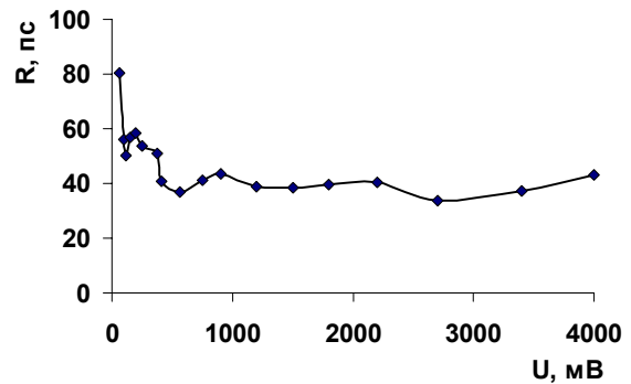
Рис. 3. Зависимость временного разрешения ФСП от входной амплитуды
