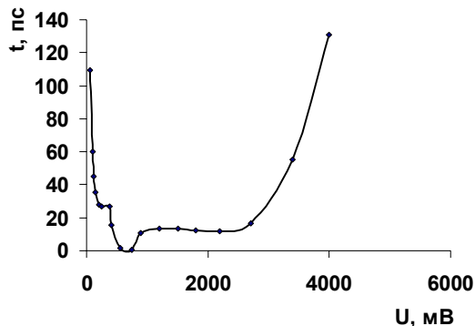
Рис. 2. Зависимость “delay walk” ФСП от входной амплитуды.
