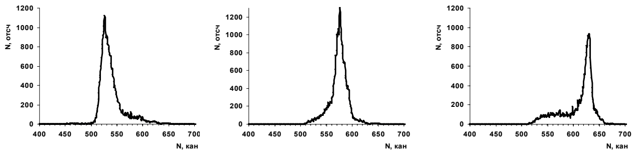
Рис. 5. Спектры временных совпадений для трех положений детектора относительно оси коллиматора.
