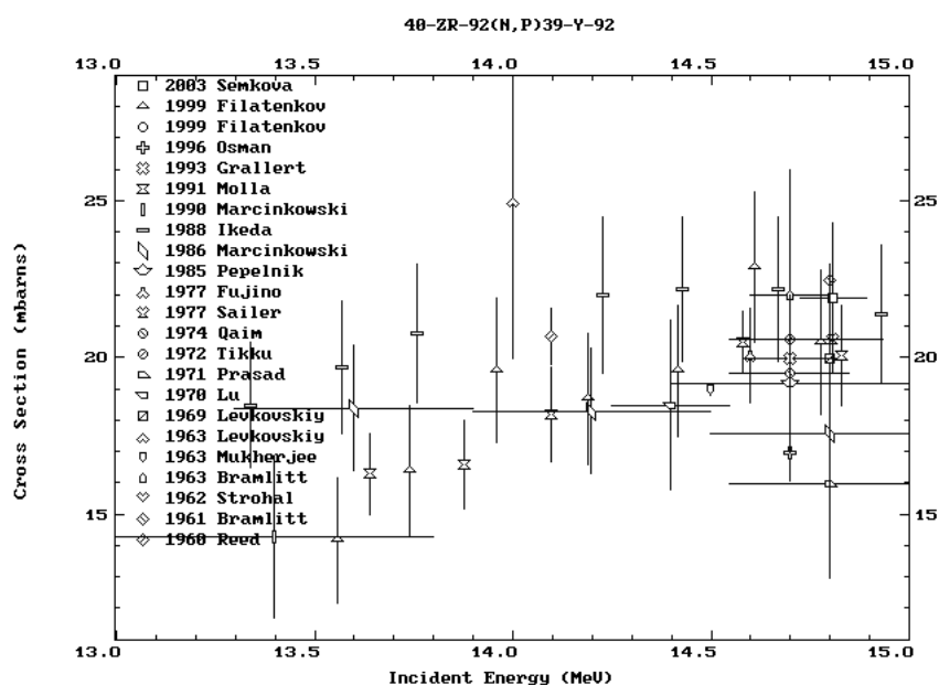
Рис. 1. Енергетична залежність перерізу ядерної реакції ^{92}\text{Zr}(n, p)^{92}\text{Y} [2].
