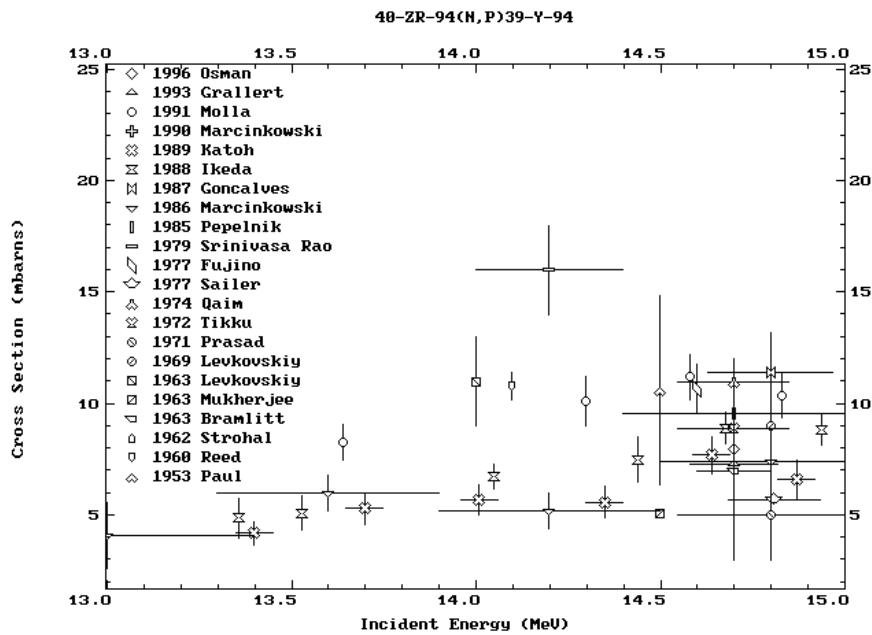
Рис. 2. Енергетична залежність перерізу ядерної реакції ^{94}\text{Zr}(n, p)^{94}\text{Y} [2].
